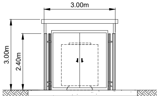
ELEVATION 'D'
